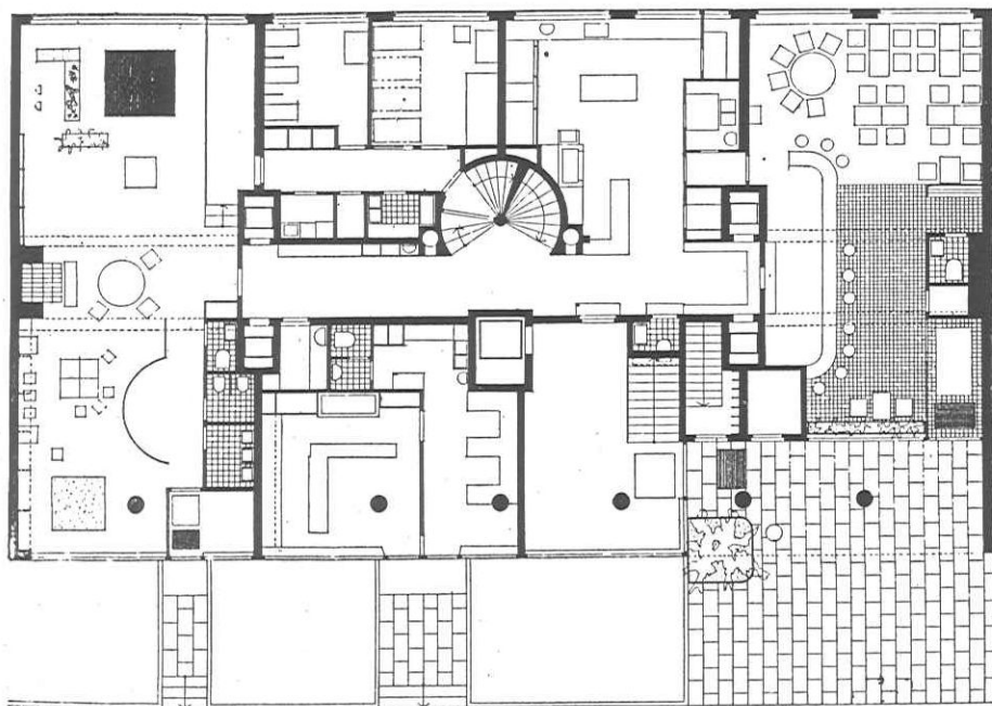
Plan av bottenvåningen.
